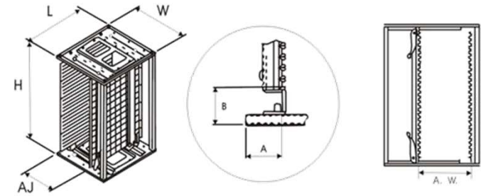
收集箱（架）尺寸示意 Magazine Dimensions
