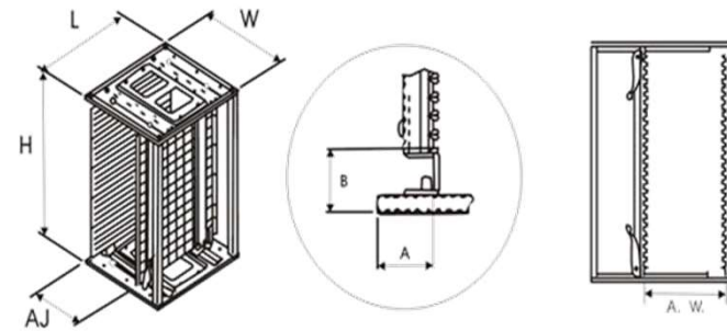
收集箱（架）尺寸示意 Magazine Dimensions
