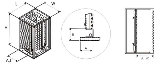
收集箱（架）尺寸示意 Magazine Dimensions
