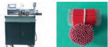
EIBC-01B - Máquina Automática de Corte, Decape e Estanhagem
