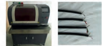
EIBC-S42 - Máquina Automática de Corte e Torção de Fio Blindado
